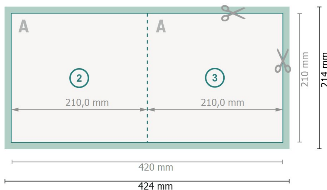
Innenseite
